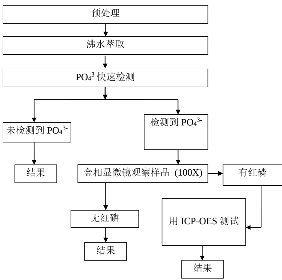
Red Phosphorus 测试流程图
