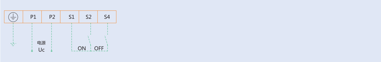
NM8（S）-100、250、630、1250电操接线图
