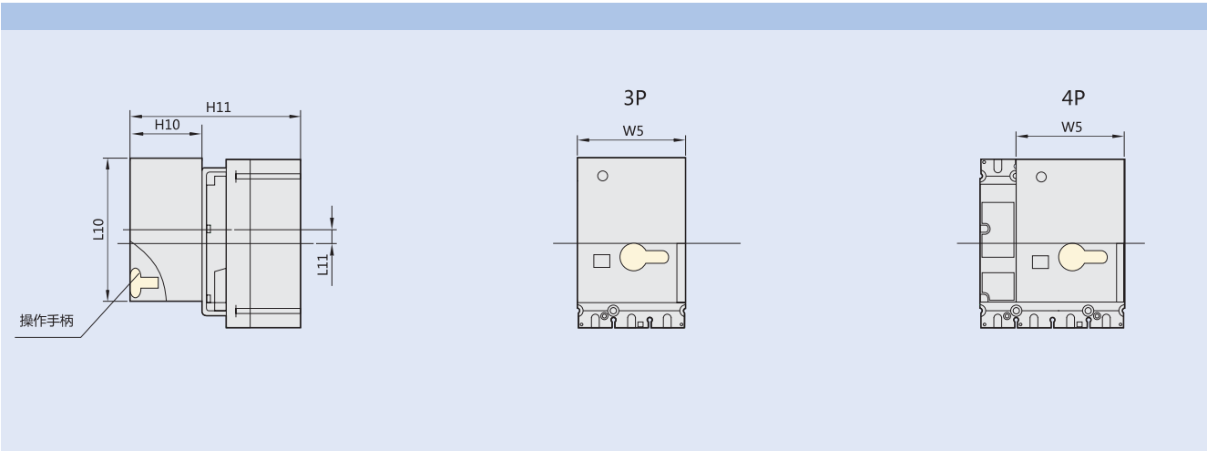
前板开孔（固定式或插入式断路器）
