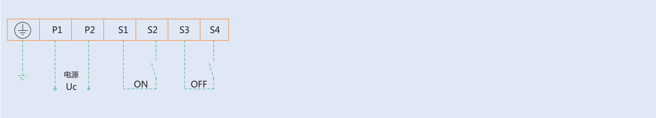
NM8（S）-800电操接线图
