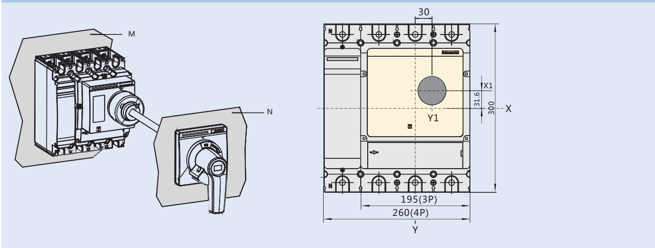
NM8S-800加长旋转手柄尺寸图
