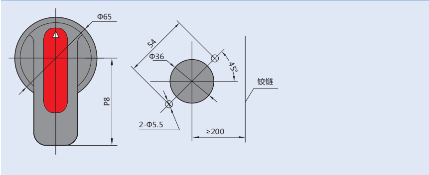
NM8(S)-100、250、630 产品手柄安装开孔示意图
