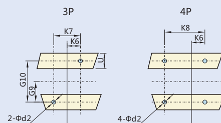
在底板 (N) 前联接
