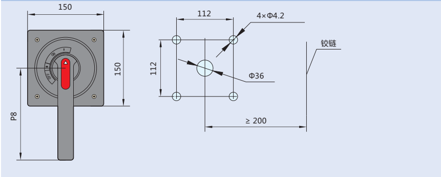
NM8(S)-1250 手柄安装开孔示意图
